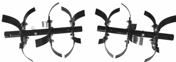
Збирання фрез
